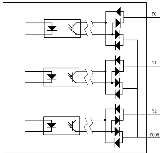
驱动器
