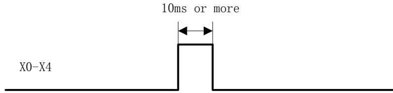
X0-X4 时序图
